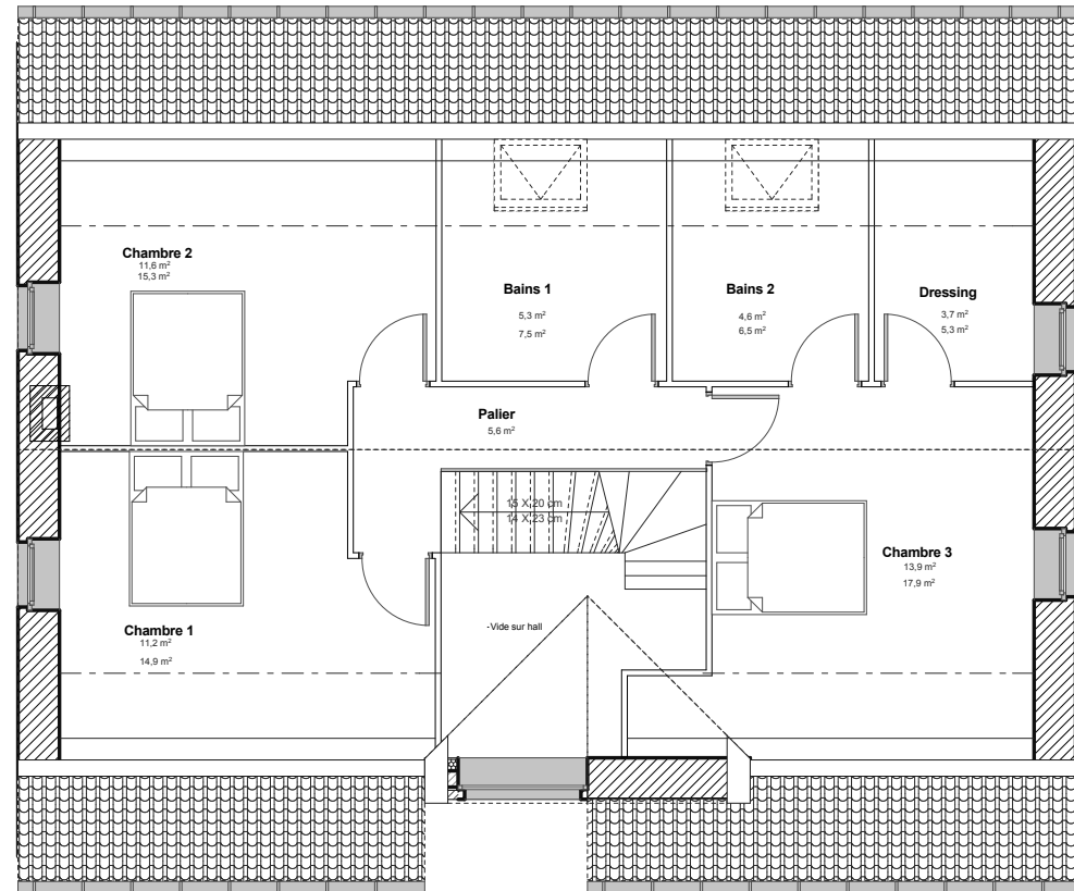
plan étage
