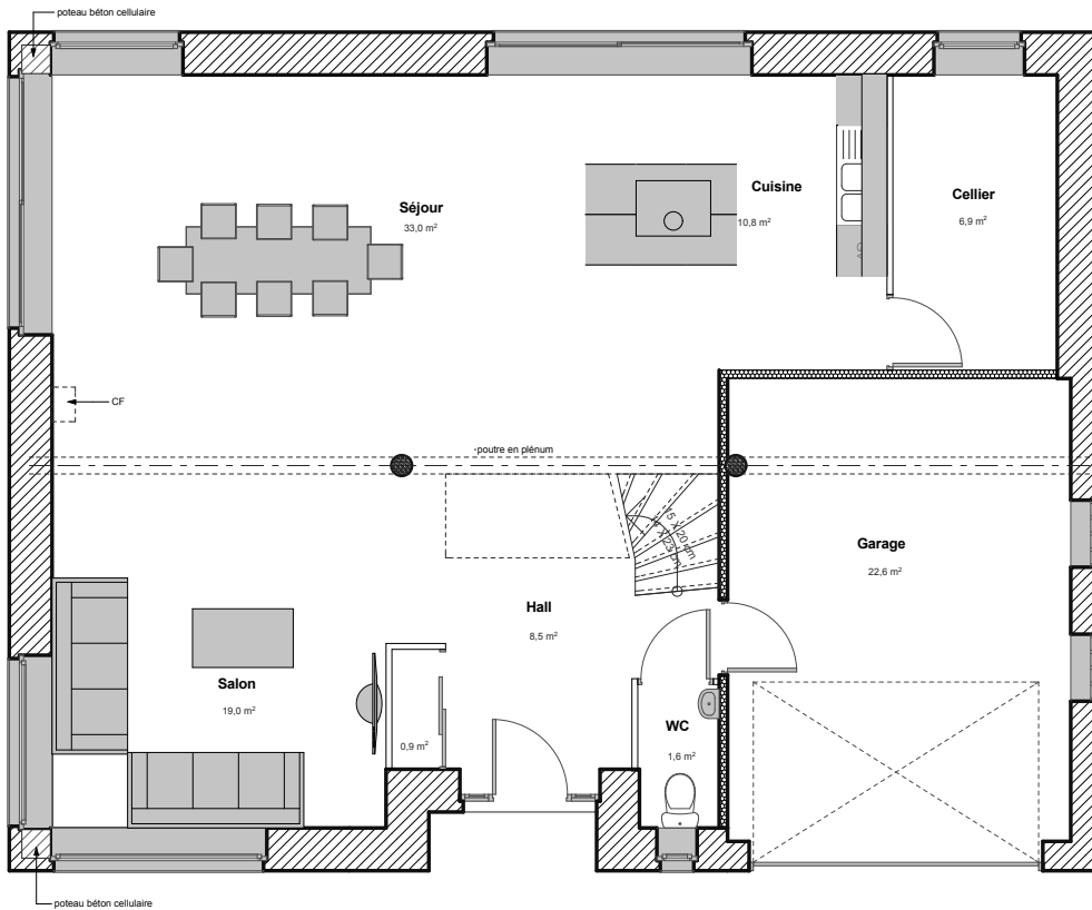
plan RDC
